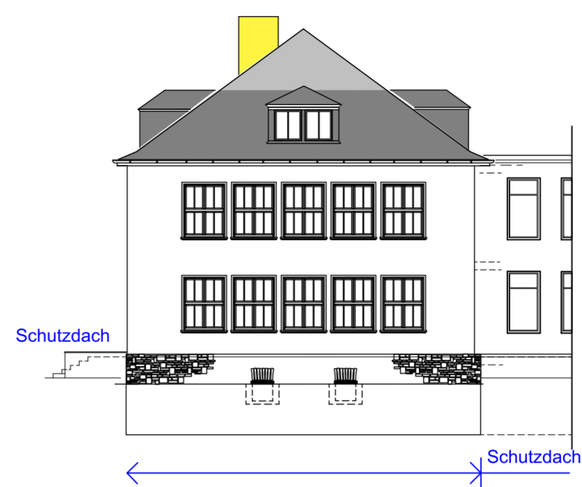
OSTANSICHT KOPFBAU
