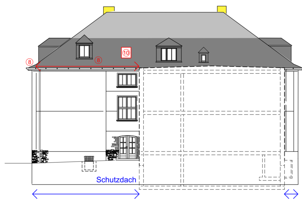
NORDANSICHT KOPFBAU
