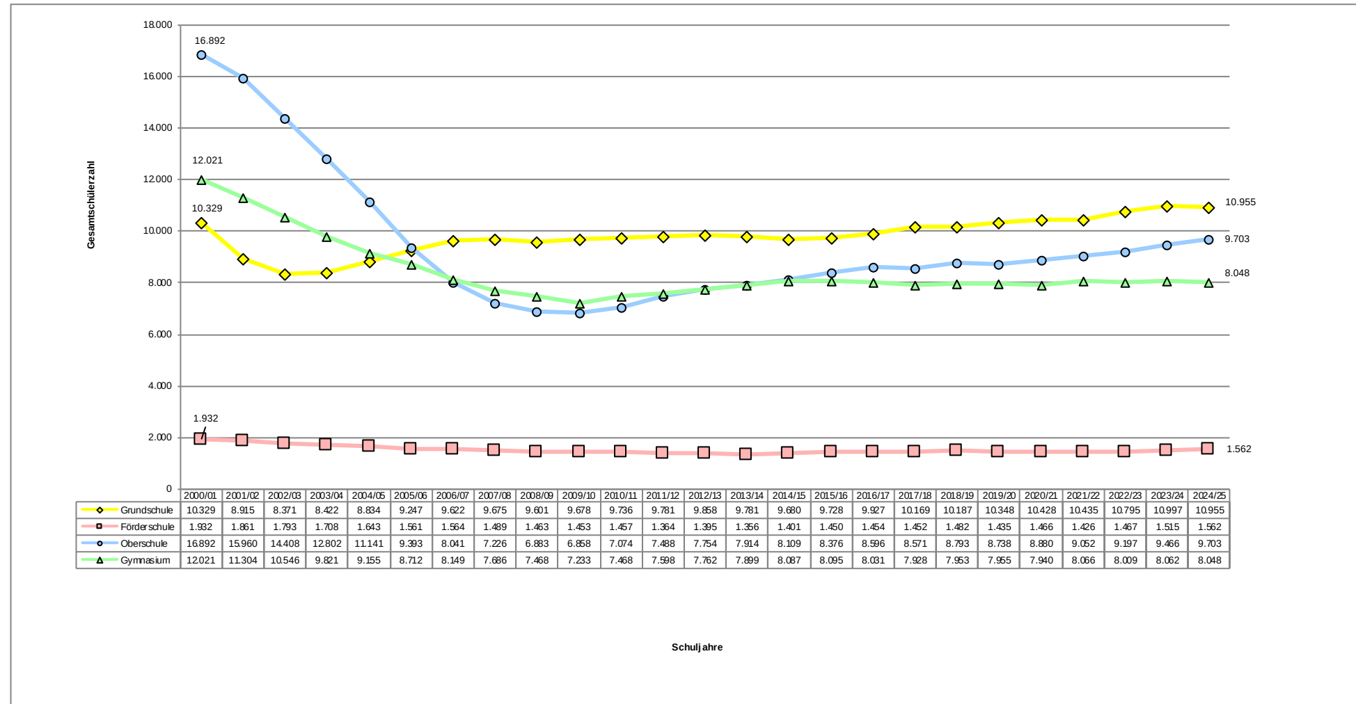
Abbildung 39: Entwicklung Gesamtschülerzahl 2000/01 – 2024/25
